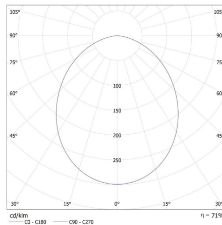
KANLUX S.A. (kat 35678) TIBERI PRO NT30W-940W / LDC (Polar)
