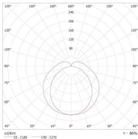
KANLUX S.A. (kat 36651) AKVO IP44 15W-NW-B S / Krzywa rozsyłu światła (biegunowo)
