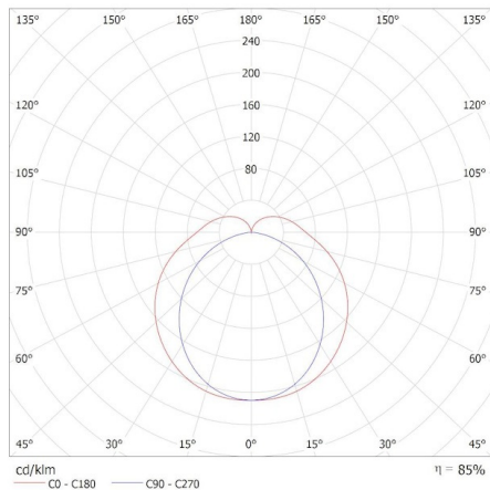
KANLUX S.A. (kat36654) AKVO IP44 20W-NW-B S / Krzywa rozsyłu światła (biegunowo)
