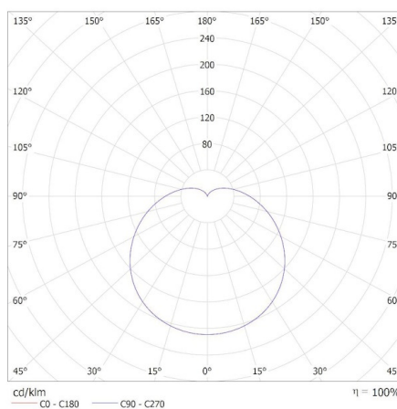
KANLUX S.A. (kat 36699) IQ-LED G45E27 5,9W-CW / Krzywa rozsyłu światła (biegunowo)
