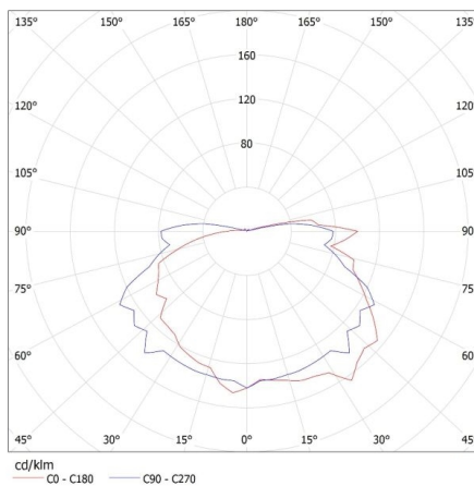
KANLUX S.A. (kat 4260) TUNA S1101 / Krzywa rozsytu światła (biegunowo)
